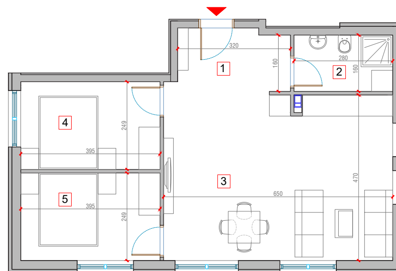
Osnova stana sa dimenzijama
